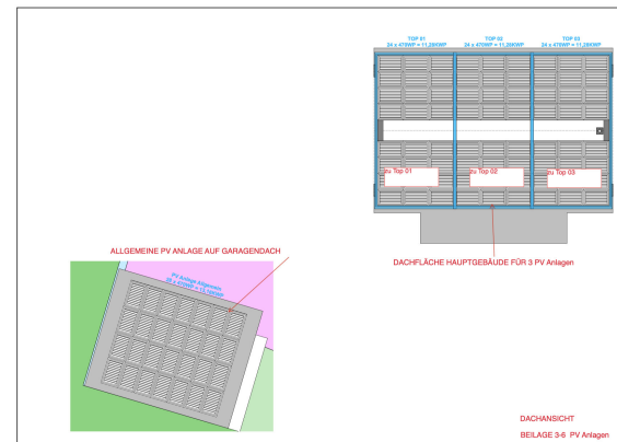
PV-Aufteilung
