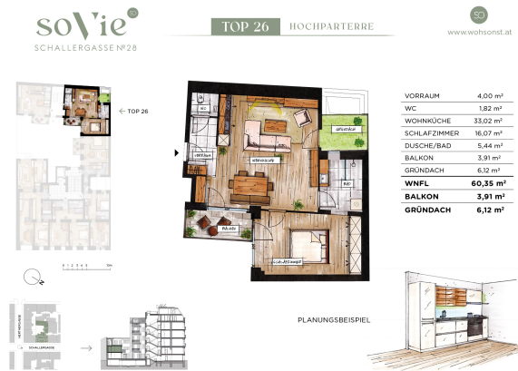
Grundriss Top26
